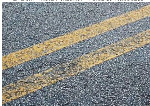
Falha em Pintura Horizontal – Perda de Visibilidade
