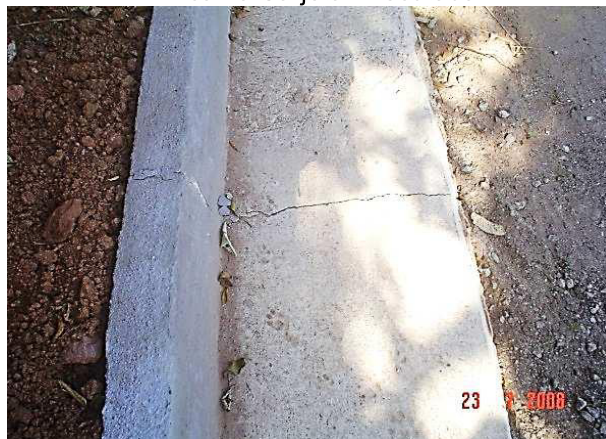
Trinca na Sarjeta Executada
